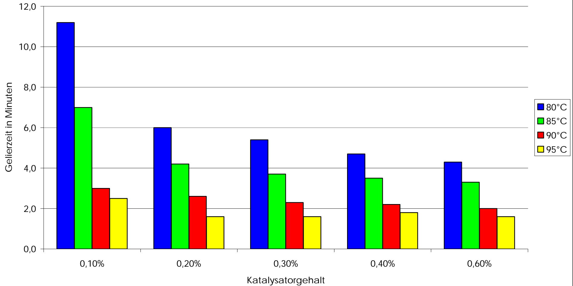
Gelierzeit von IM4500 in Abhängigkeit von Katalysatorkonz. und Temperatur (entgast)
