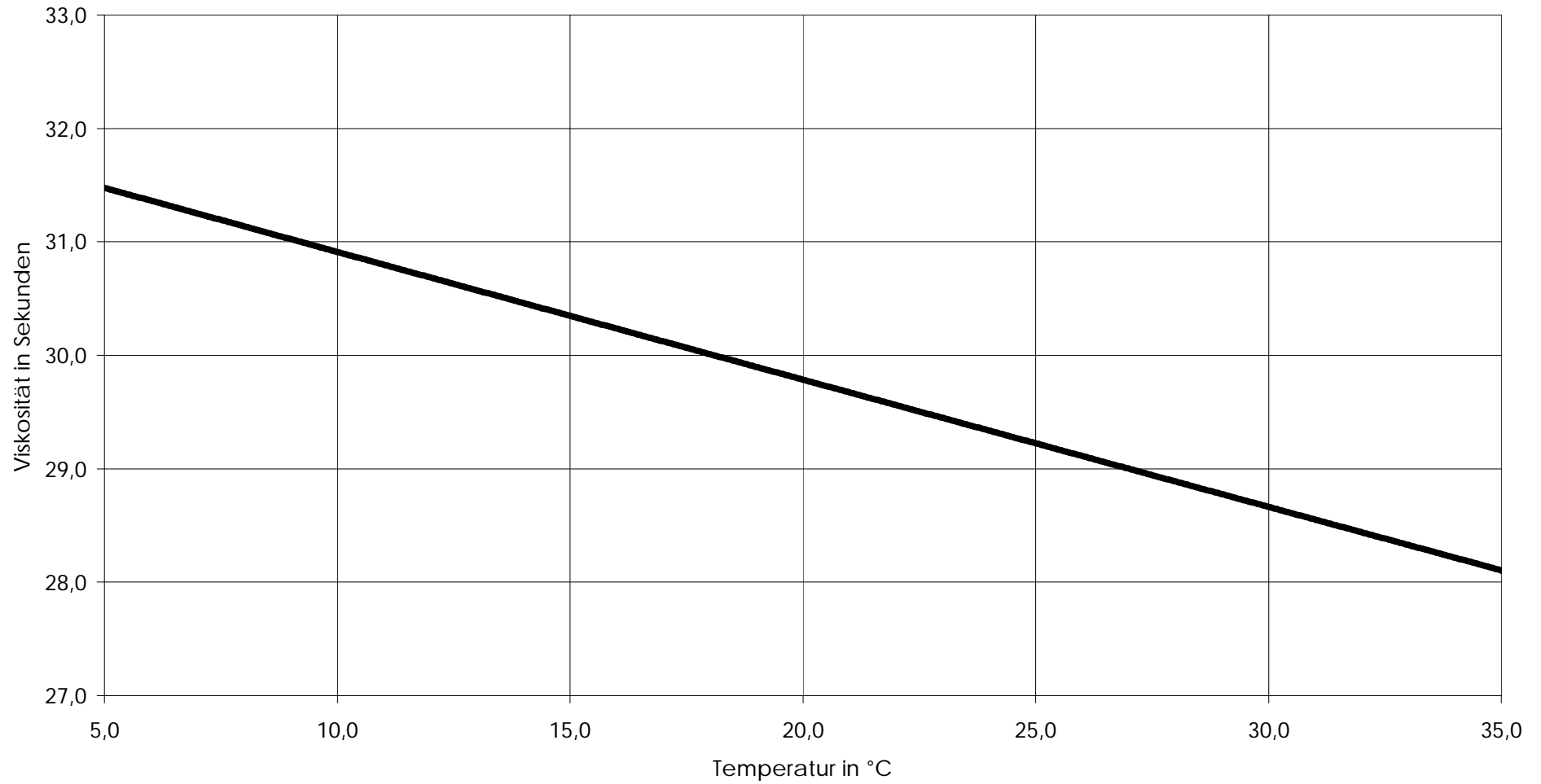
Viskosität von IM4500 bei verschiedenen Temperaturen (Zahn Cup No 1)
